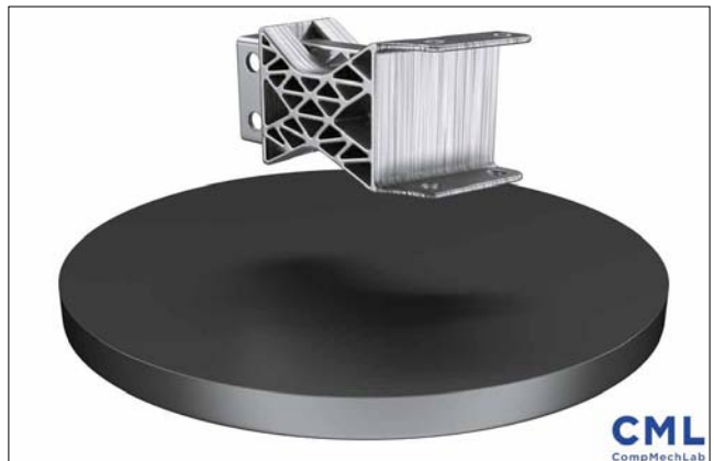
Рис. 10. Краш-бокс – устройство, поглощающее энергию при столкновении
